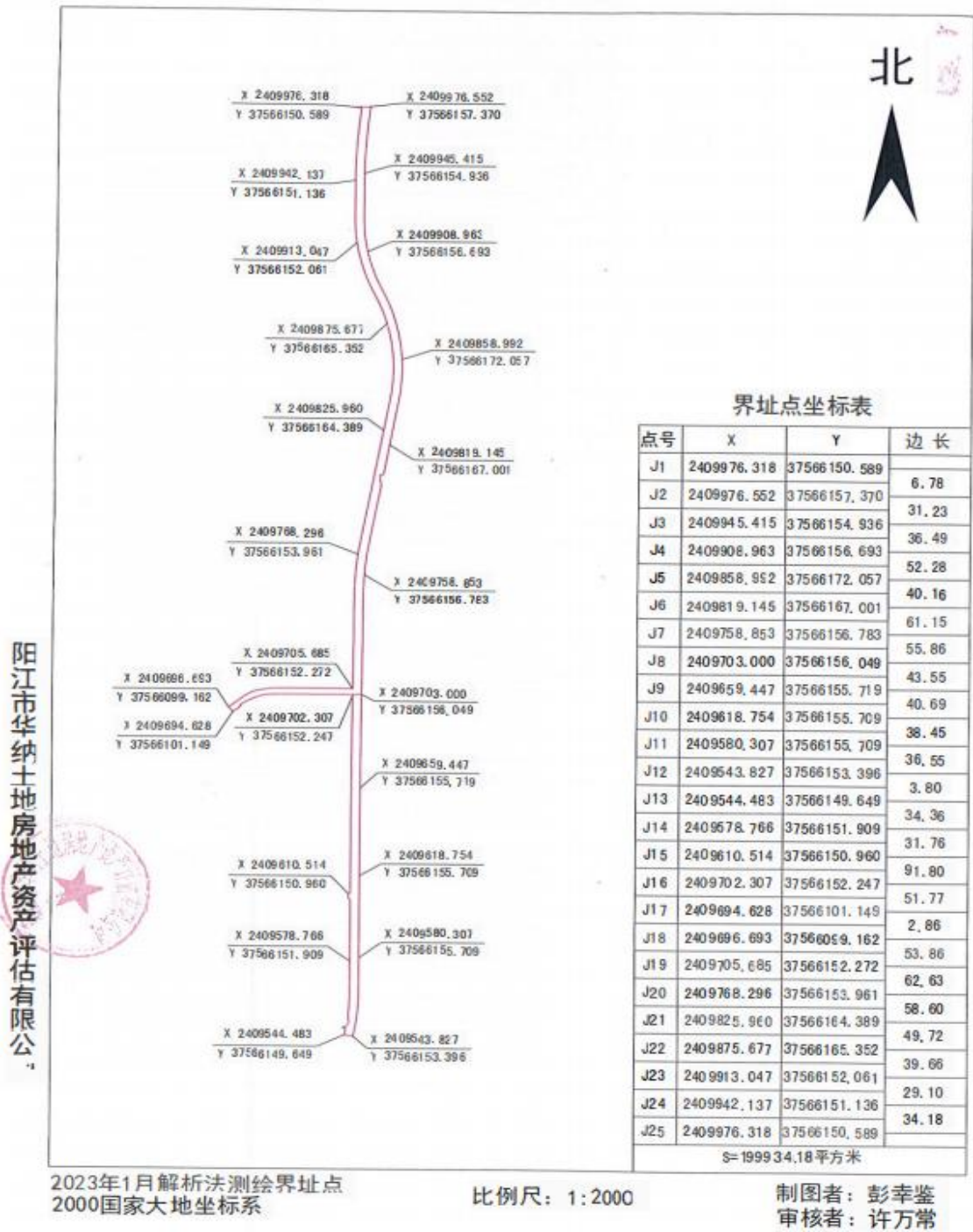
阳西县2020年度第十一批次城镇建设用地红线范围图
